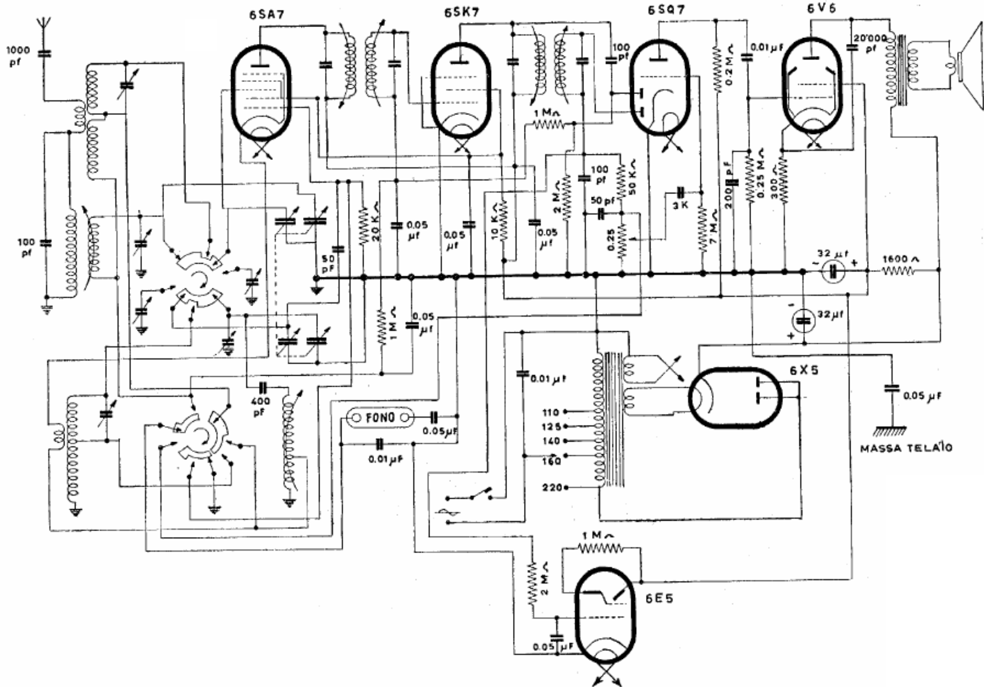
IRRADIO - Mod. E31, E35 ed E41. Onde medie e due bande onde corte. Media frequenza 467 kc/s. Potenza indistorta di uscita 3 watt. Consumo 35 watt.
